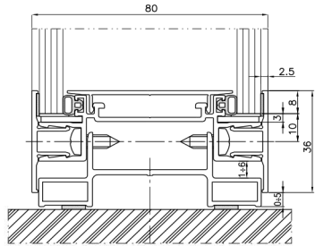
Сечение по нижней перекладине
