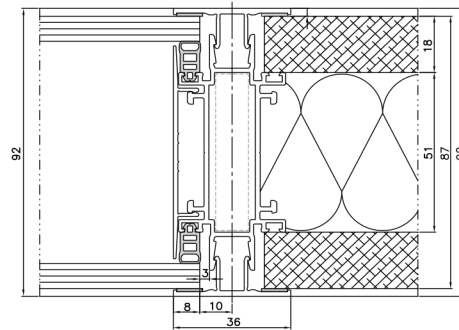
Вертикальное сечение по перегородке 92 мм
