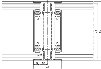
Вертикальное сечение по перегородке 80 мм
