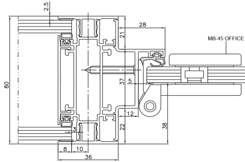
Горизонтальное сечение дверей
