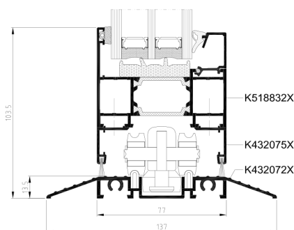
Нижнее сечение дверей с низким порогом
