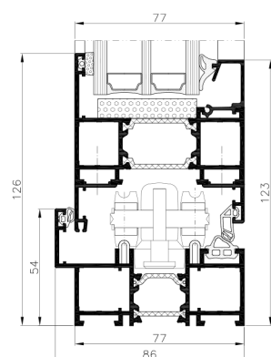
Нижнее сечение дверей с уплотнительной прокладкой притвора
