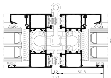
Сечение через соединение створок дверей
